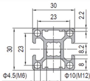
30x30 2 slots Type B
