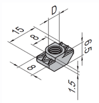
T Nut-8-M4 T Nut-8-M5 T Nut-8-M6
