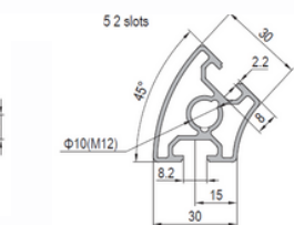
30x30 R45 2 slots
