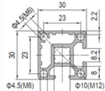
30x30 2 slots Type A
