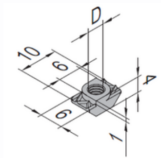
T Nut-8-M4 T Nut-8-M5 T Nut-8-M6
