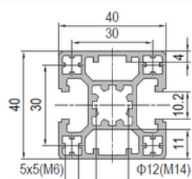
40x40 2 slots Type B
