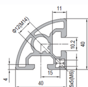
40x40 R90 2 slots
