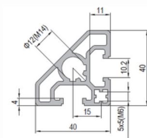
40x40 T45 2 slots
